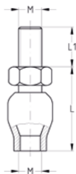
Rotule de suspension courte
