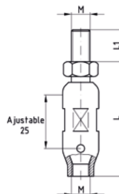
Rotule de suspension longue
